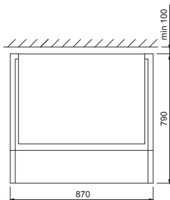
Boven aanzicht
